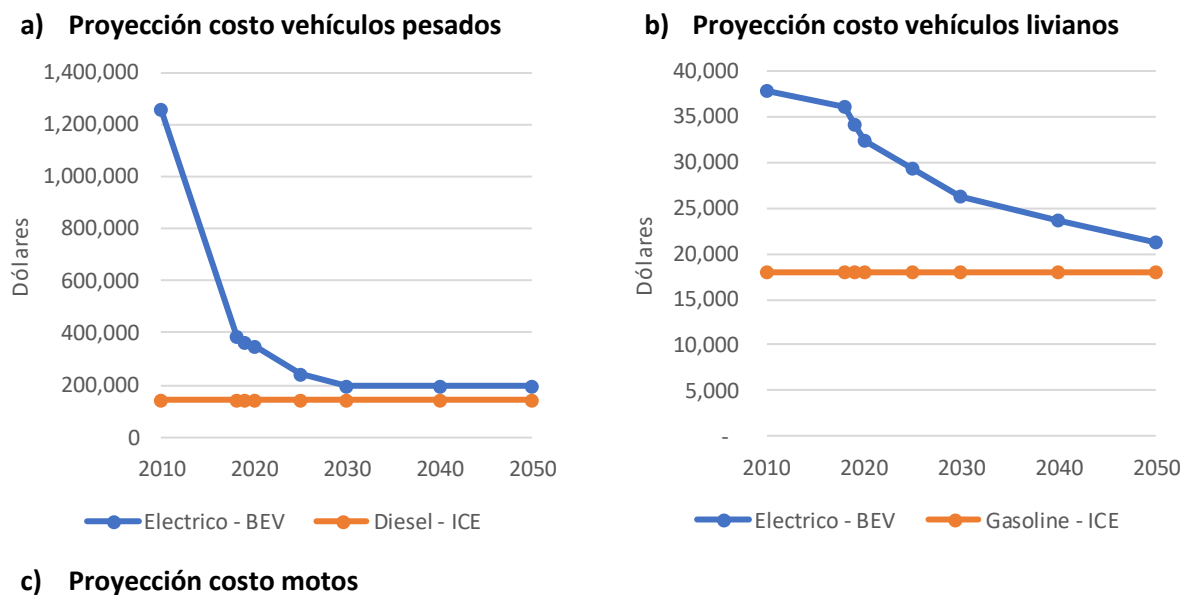
Figura 6-10: Proyección de costos de vehículos eléctricos hasta 2050, comparados con costos vehículos de combustión interna
