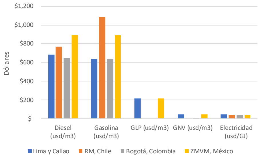
Figura 6-11: Costos combustibles y electricidad utilizados en HETRANS
