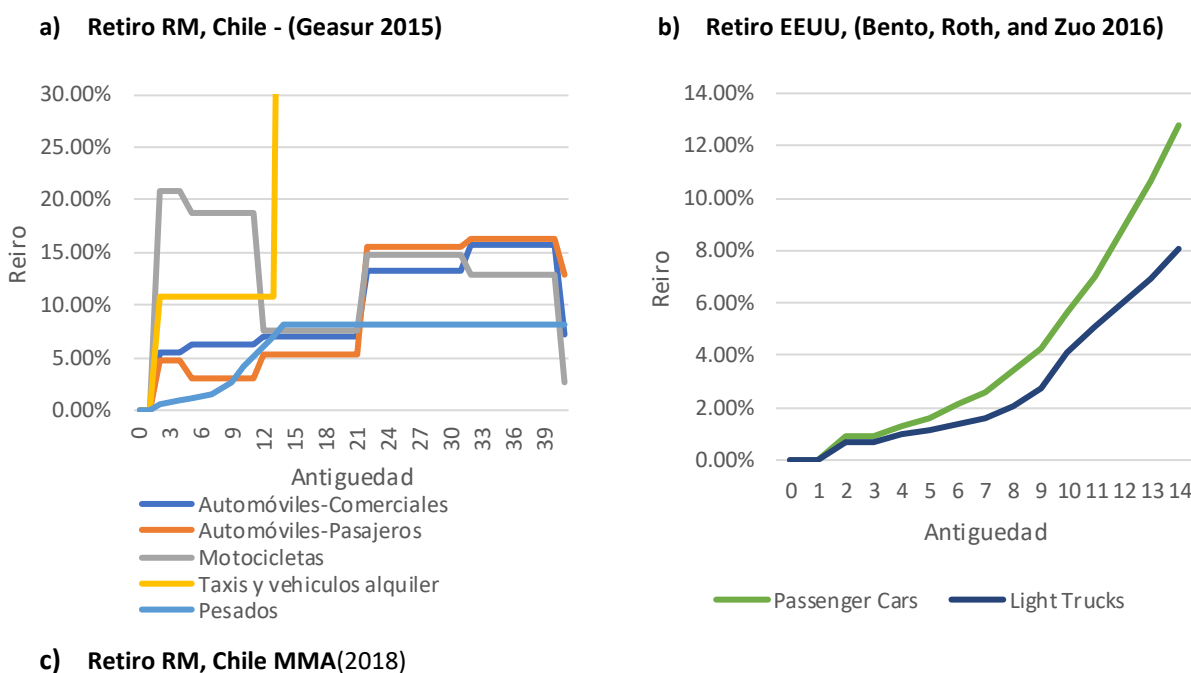
Figura 6-6: Curvas de retiro disponibles en HETRANS.
